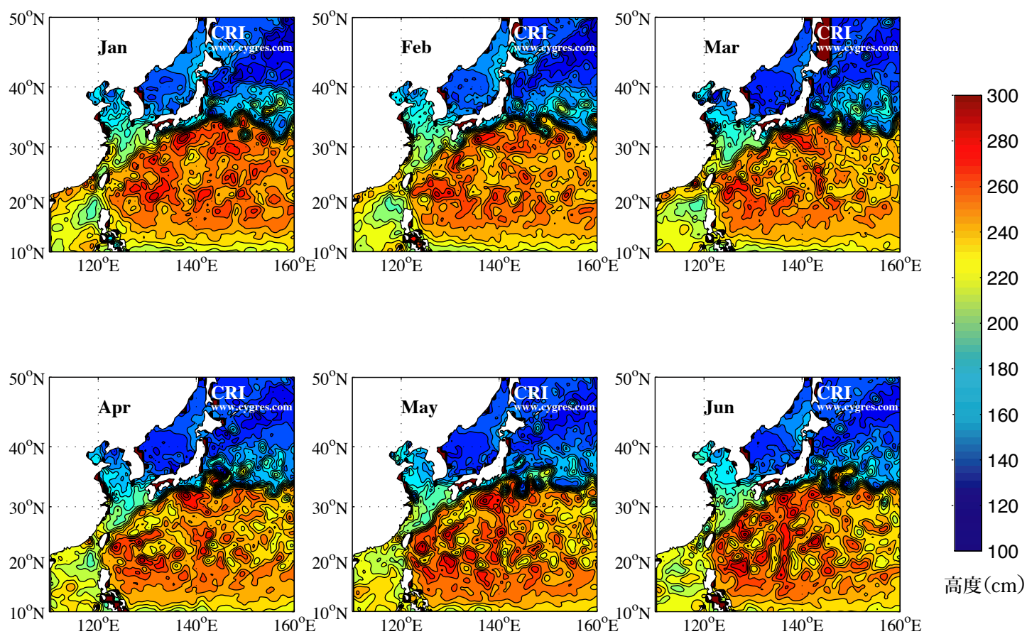
月平均海面高度(2006年1月~6月)
